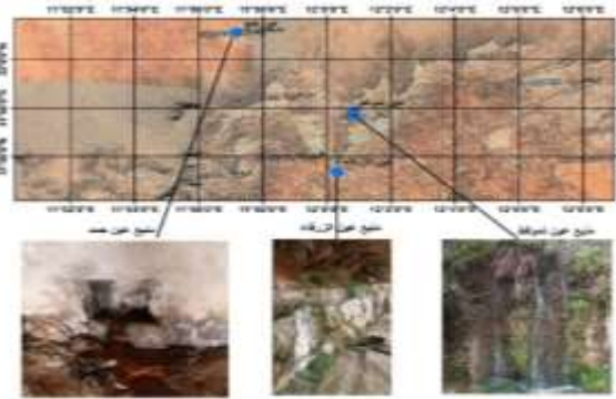
شكل 3. مواقع الينابيع المائية بمنطقة الدراسة "مدينة جادو"
