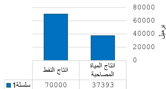
شكل 1. كميات المياه المصاحبة المنتجة، وكميات النفط المنتج بحقل النافورة على أساس يومي خلال شهر يناير 2017 م [2]
