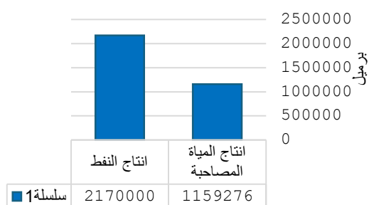
شكل 1. كميات المياه المصاحبة المنتجة، وكميات النفط المنتج بحقل النافورة على أساس شهري خلال شهر يناير 2017 م [2]
