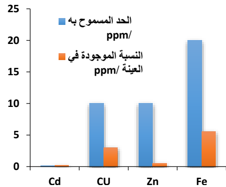
الشكل 2. يوضح العناصر الثقيلة المتمثلة في الكاديوم والنحاس والزنك والحديد للعينة A 2 حيث نلاحظ ان كل النسب في المستوي المسموح بها
