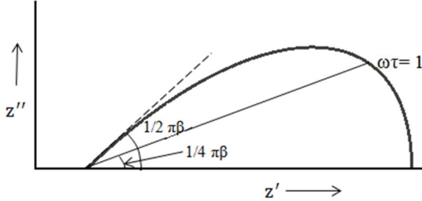
شكل 2. مخطط المعاوقة لمعادلة كول- دافيدسون بين الجزء التخيلي Z'' والجزء الحقيقي Z' .
