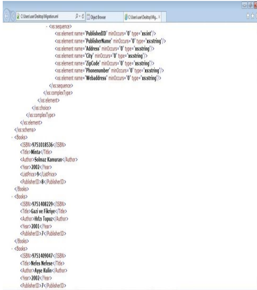
Fig. 7. An XML document.
