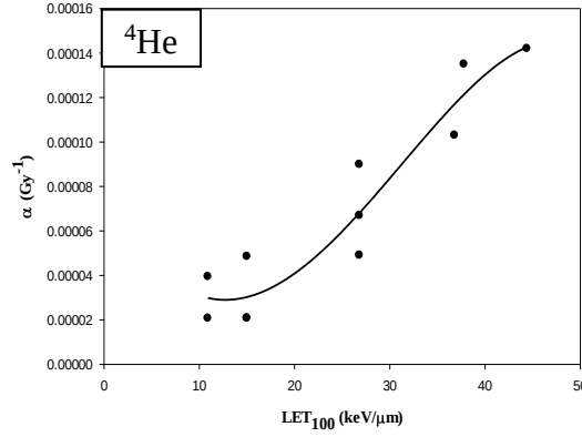
شكل 3. العلاقة بين بارامتر الحساسية الإشعاعية للطفرة الجينية ( \alpha (Gy -1 ) وبارامتر الطاقة الخطية المنتقلة المقيدة LET 100 (keV/μm) لجسيمات ألفا.
