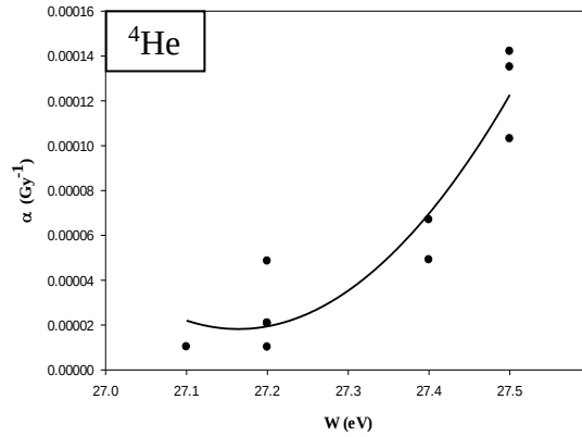
شكل 4. العلاقة بين بارامتر الحساسية الإشعاعية للطفرة الجينية ( \alpha (Gy -1 ) وبارامتر متوسط الطاقة W(eV) لجسيمات ألفا.
