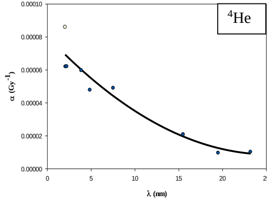
شكل 5. العلاقة بين بارامتر الحساسية الإشعاعية للطفرة الجينية ( \alpha ( Gy^{-1} ) وبارامتر متوسط المسار الحر \lambda (nm) لجسيمات ألفا.
