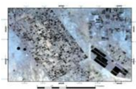
a-Landsat image -2006
