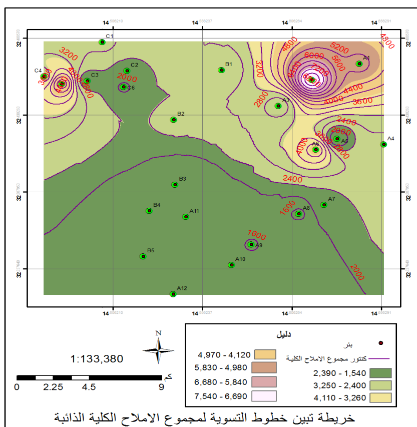
شكل 2. التوزيع المكاني للأملاح الكلية الذائبة (TDS).
