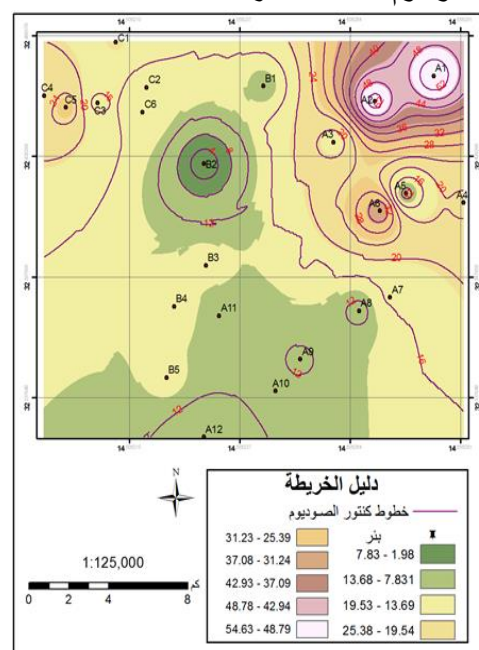
شكل 3. التوزيع المكاني لتركيز الصوديوم ( Na^{+} )
