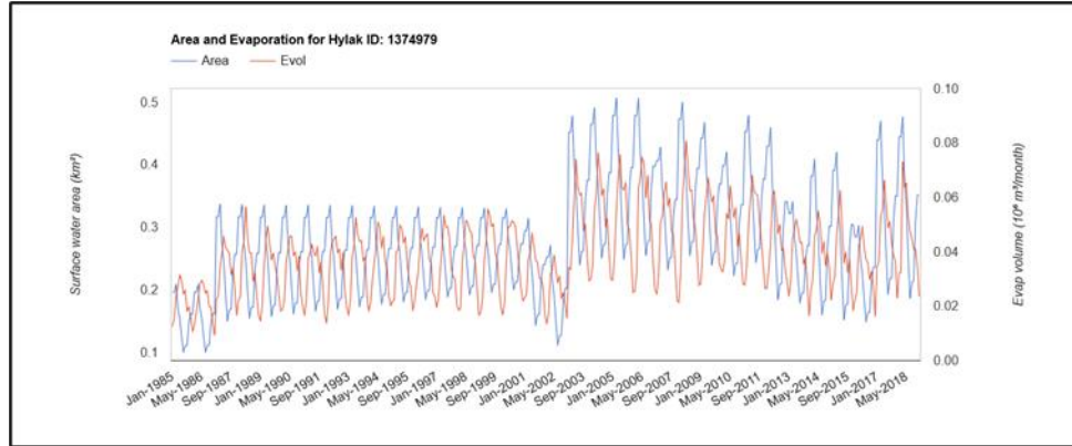
شكل 4. معدل البخر الشهري والمساحات السطحية للمياه في سد وادي غان
