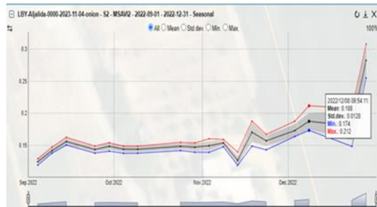
شكل 2: قيم مؤشر الغطاء النباتي المعدل للتربة جدول 1: بعض قيم MSAVI حتى وصوله 0.212
