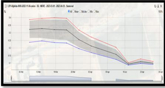
شكل4: قيم مؤشر الاختلاف الطبيعي للحافة الحمراء ولمراقبة رطوبة التربة والمحصول تم استخدام مؤشر الجفاف ( Normalized Multi-band Drought Index ) (NMDI) من بداية ظهور النبات حتى جني المحصول، وكانت القيم المتحصل عليها في تزايد، مما دل على عدم تعرض النبات لأي إجهاد مائي شكل(5) ( Zhour (NAJOUIL,2020).
