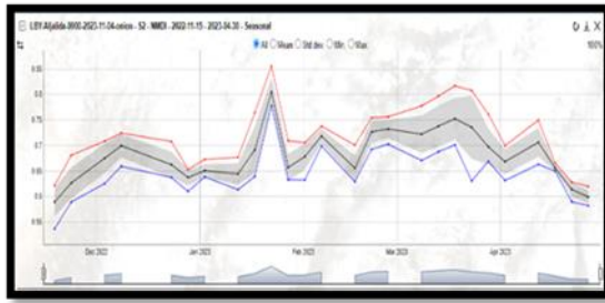
شكل5: قيم مؤشر NMDI من منصة المسبار وقد لوحظ وجود قيم متطرفة في قيم كل المؤشرات المختارة، وعند الرجوع إلى صور الأقمار الصناعية في تواريخ هذه القيم اتضح أن هذه القيم ما هي إلا نتيجة لوجود السحب الكثيفة، وفي بعض الأحيان كان السبب هو ظل السحب الذي أثر على هذه القيم شكل(6).
