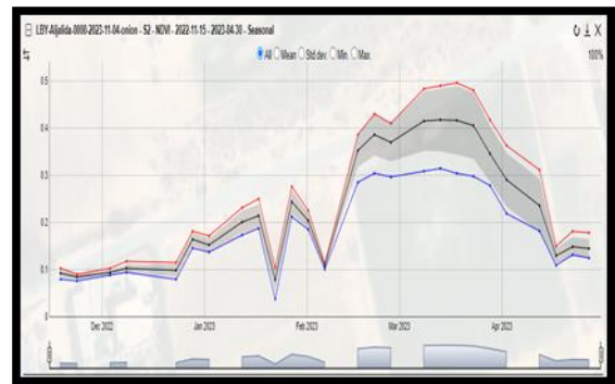
شكل3: قيم مؤشر الاختلاف الطبيعي للغطاء النباتي
