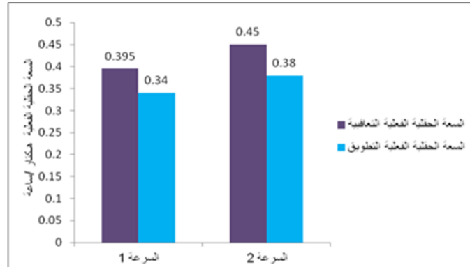
شكل 1. تأثير السرعة وطريقة الدخول إلى الحقل على السعة الحقلية الفعلية.
