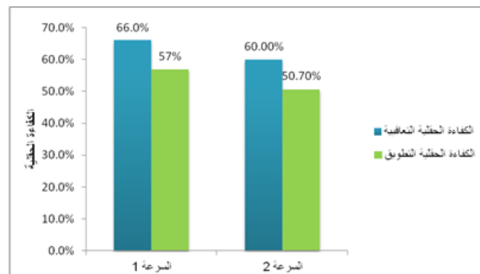
شكل 3. تأثير طريقة الدخول للحقل على الكفاءة الحقلية.
